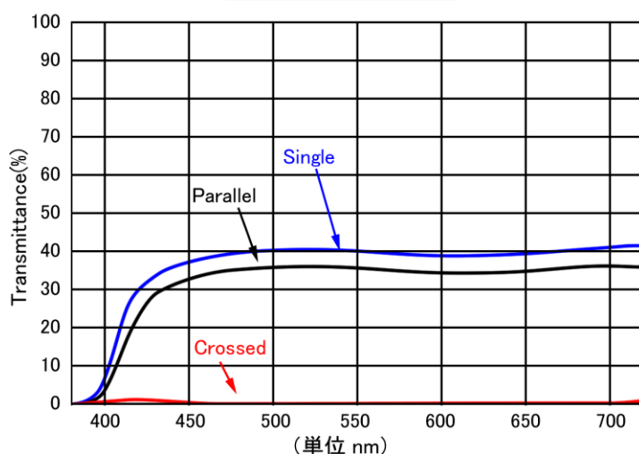
MLPH40 分光透過率特性
